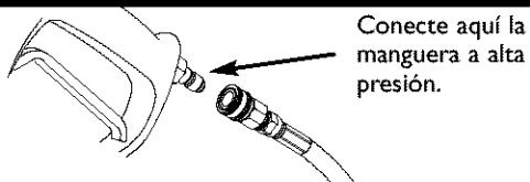
Figura 12 - Conecte la Manguera a alta Presión a la Pistola Rociadora
